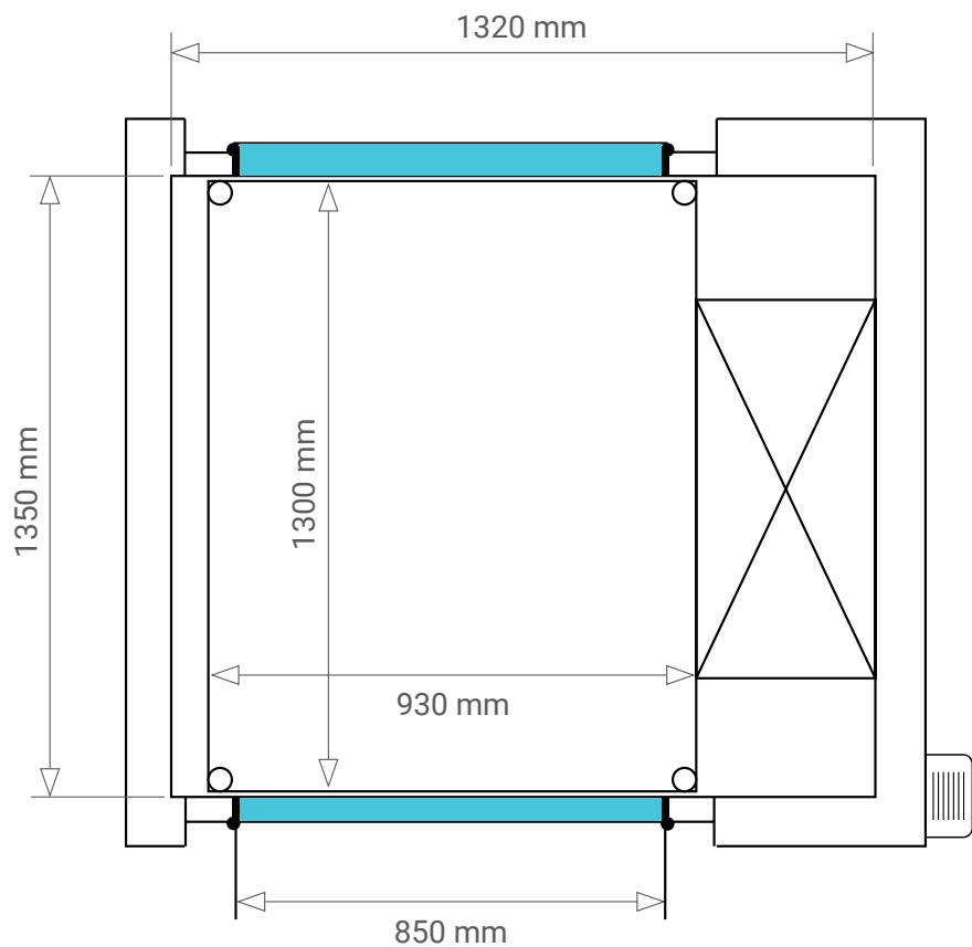
Control Box: 256mm (W) x 168mm (D) x 1982mm (H)
